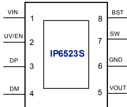
图 2 IP6523S 引脚图
